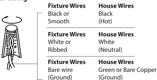
Fig.3 Wiring
